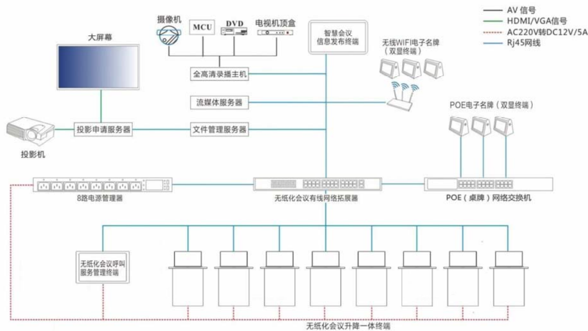
智能无纸化会议系统原理图
